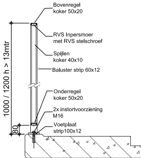
Doorsnede A-A
