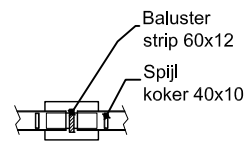
Doorsnede B-B
